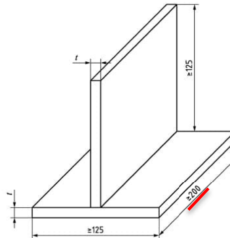
Kuva 4 Levykoekappaleen mitat pienihitsauksessa
