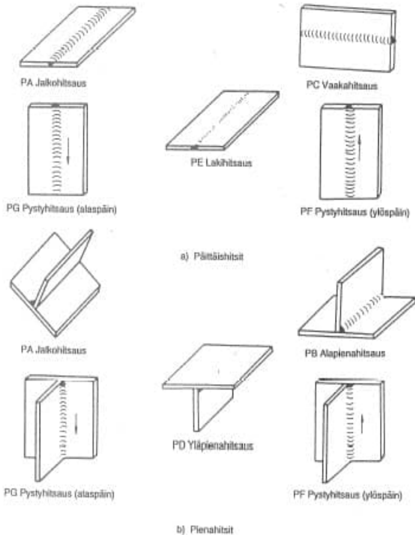
Kuva 1 Läpähitsauksen asennot
