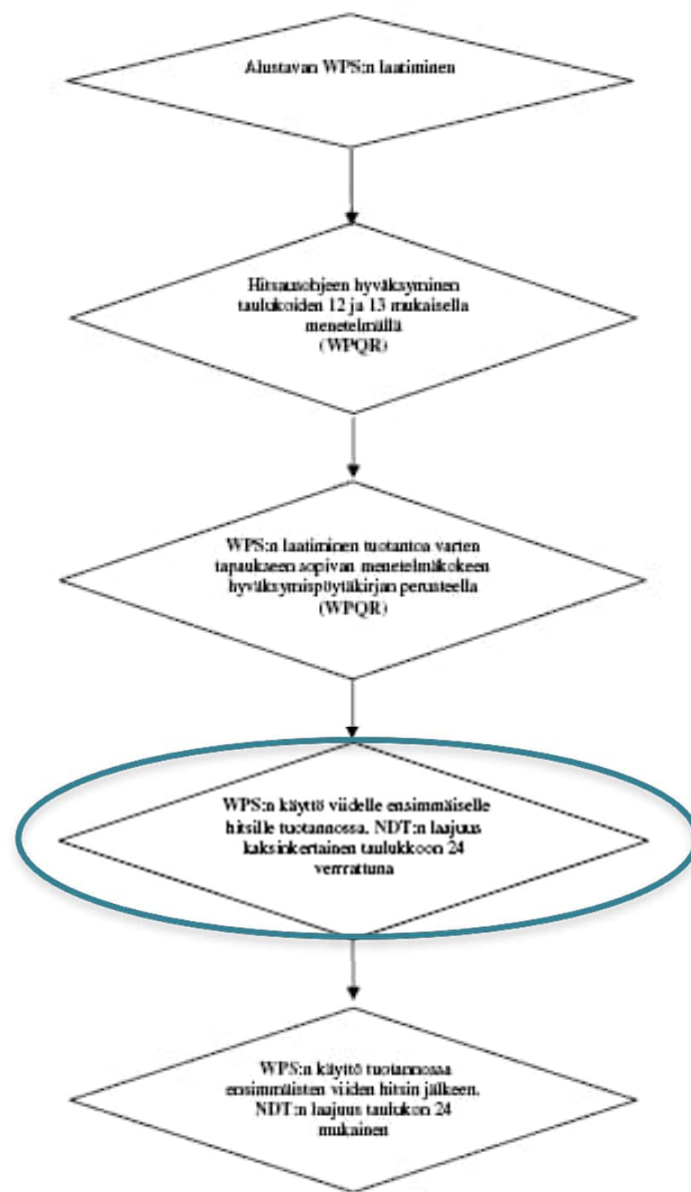
Kuva L.1 Lohkokaavio WPS:n laadintaan ja käyttöön
