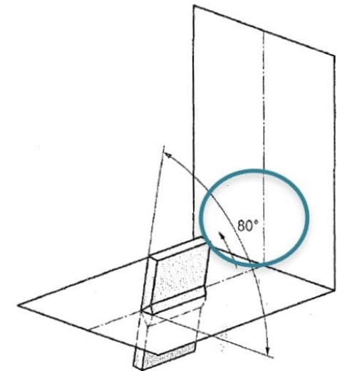
Kuva A.11 Lakiasento (PE) kiiltevuusto leranssi
