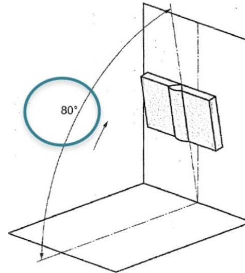
Kuva A.10 Lakiasento (PE) kiiltevuusto leranssi
