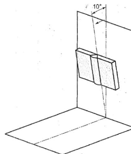
Kuva A.13 Pysiasento (PF, PG) kaltevuustoleranssi
