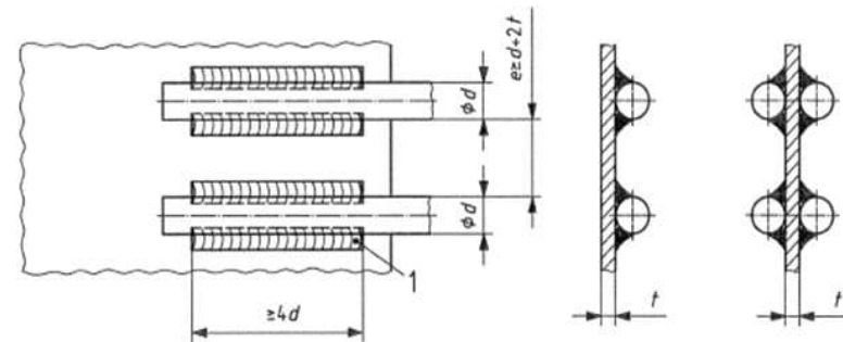
b) Kahdelta puolelta hitsattu kylkiliitos
