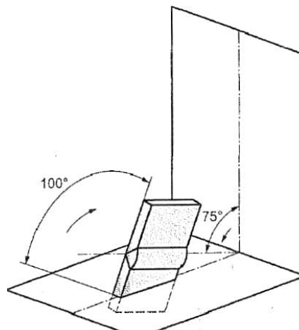
Kuva A.15 Pysiasento (PF, PG) kaltevuustoleranssi ja kiiltevuustoleranssi
