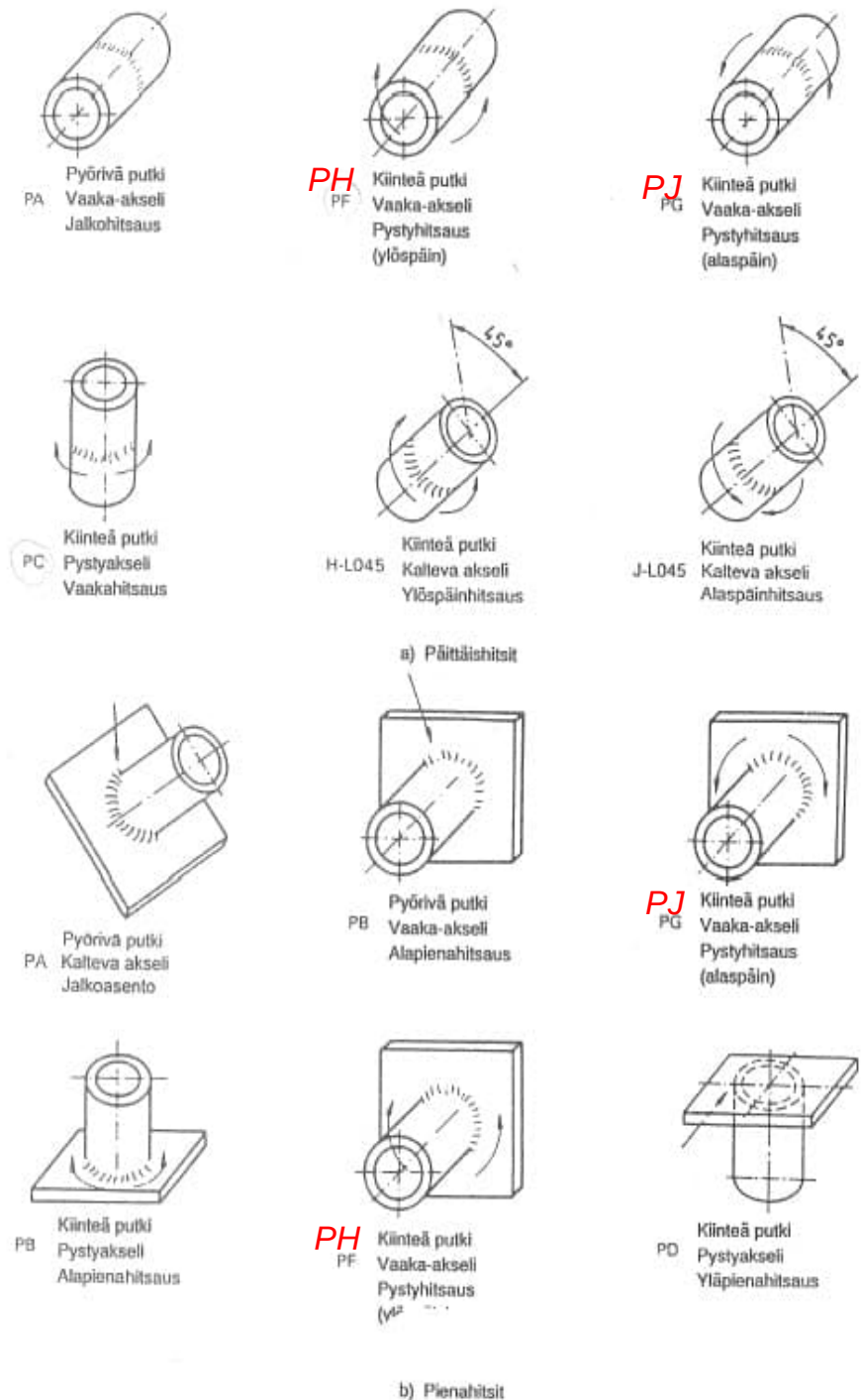
Kuva 2 Putkihitsauksen asennot
