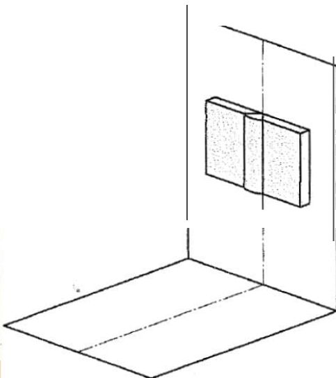
Kuva A.12 Perusasento (PF, PG)
