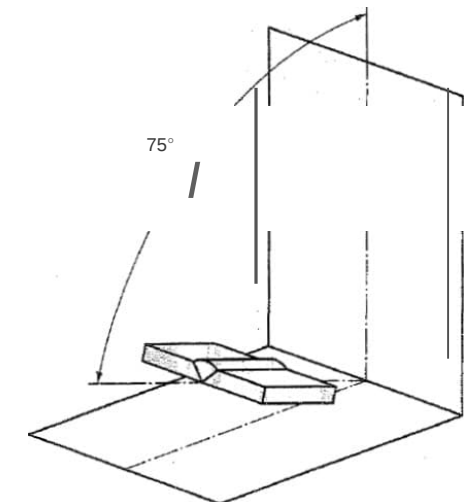
Kuva A.14 Pysiasento (PF, PG) kaltevuustoleranssi
