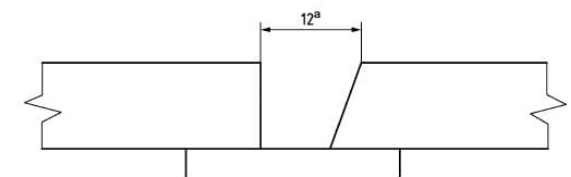
Kuva C.1 Yhdistetty FW/BW koekappale
