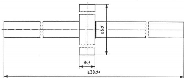
Kuva C.2 Limiliitoksen koekappale (vetokoe)
