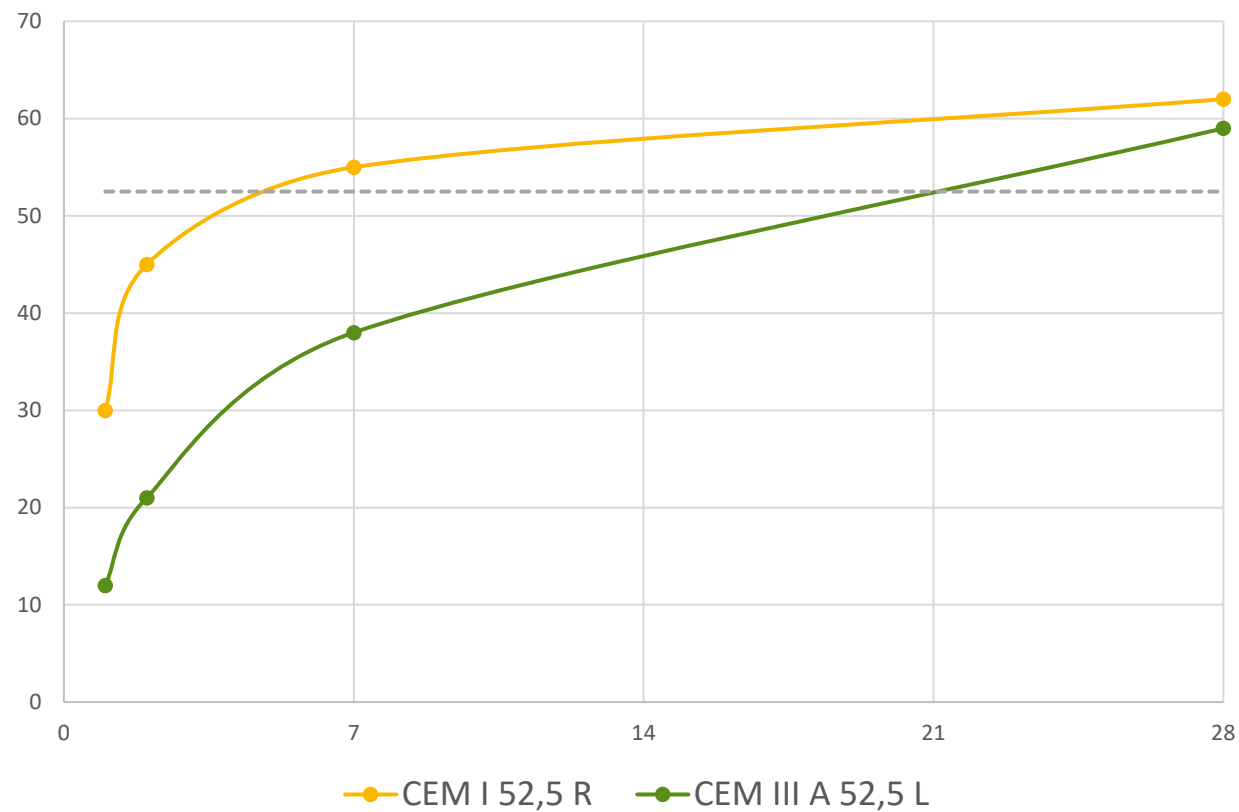
Lujuusluokat 52,5 R ja 52,5 L
