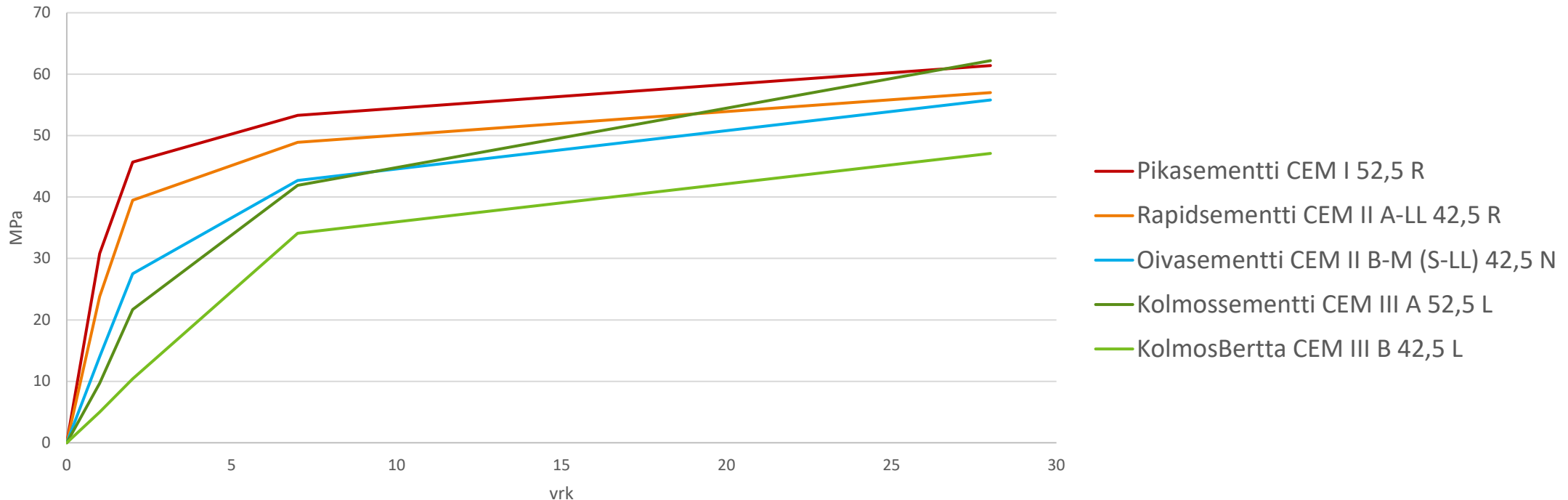
Sementtien prismalujuudet (v/s-suhde 0,50)
